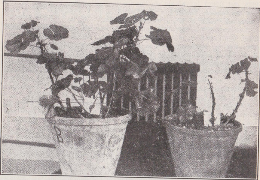
FIG. 7. — Aspect des géraniums au 17 novembre 1928. La plante portant le « circuit ouvert » est en excellente condition de végétation. Au contraire, la plante témoin voisine apparaît dans un état misérable. Sur la première, on aperçoit nettement le germe portant la tumeur desséchée; sur la seconde, le germe portant la tumeur non encore morte et qui n'a pas beaucoup grandi.
